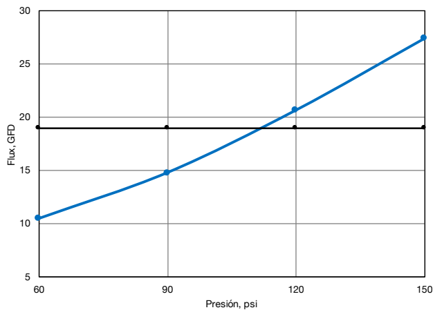
Figura 3. Flux vs Presión A condiciones de laboratorio se alcanza un flux de 19 GFD (Gal/ft 2 -día) a 110 psi. Este flux es el máximo recomendado para agua de pozo.
