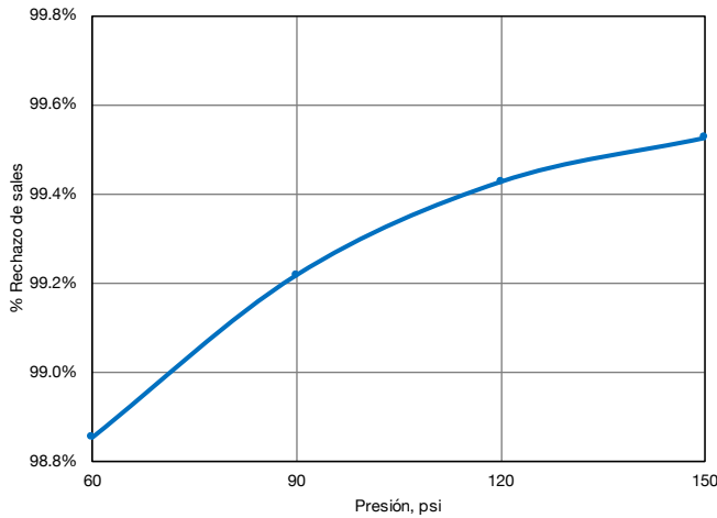
Figura 1. Rechazo de sales vs Presión A condiciones de laboratorio se obtiene un rechazo de sales de 99.4% a 110 psi. Para 2,000 mg/l de sales disueltas en la entrada, el permeado tendrá una calidad de 12 mg/l.
