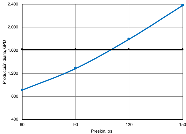
Figura 2. Producción diaria vs Presión A condiciones de laboratorio se obtiene una producción de 1,600 GPD a un flux de 19 GFD (Gal/ft 2 -día) a 110 psi.
